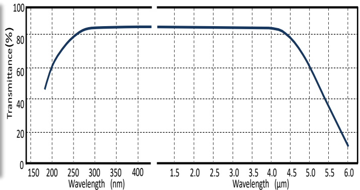
【サファイア透過率 (Transmittance)】
